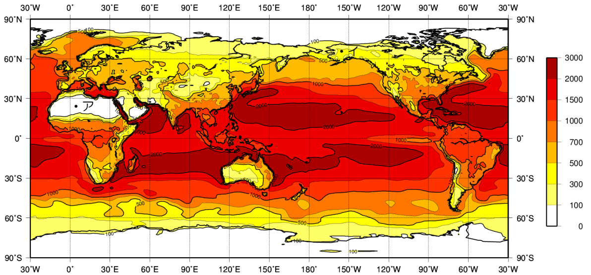
図1 世界の年蒸発散量 (陸域) と年蒸発量 (海洋) の分布 (提供: 気象庁)
