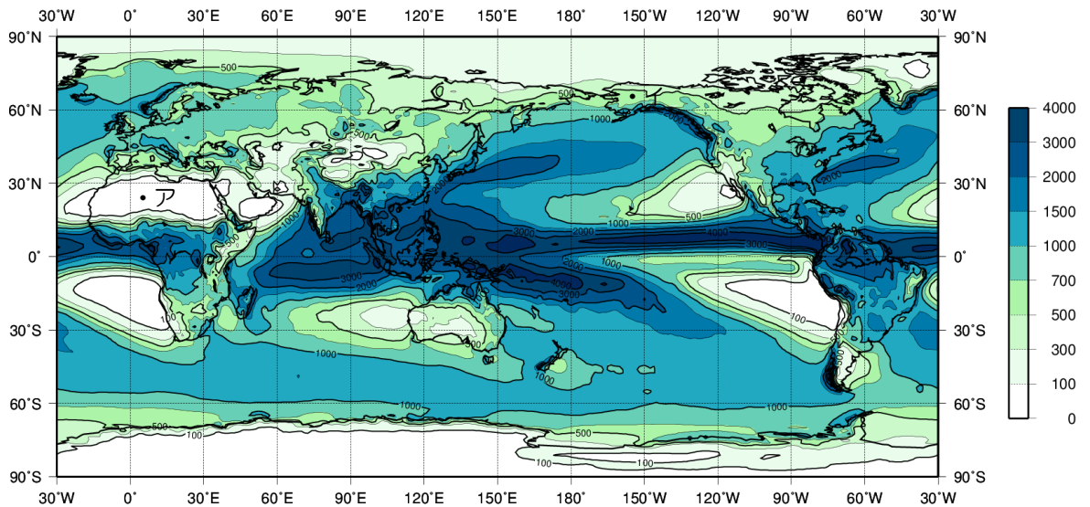
図2 世界の年降水量の分布 (提供: 気象庁)
